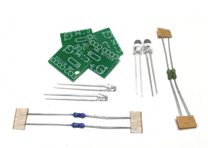
Einzelteile des IR-Sensors für 2 Spuren
