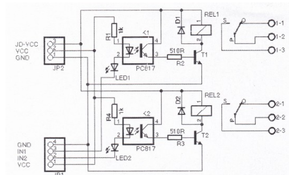
Relais-Modul (2 Kanal)
